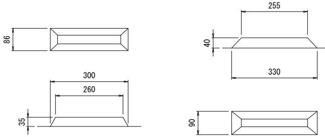
凸部詳細
